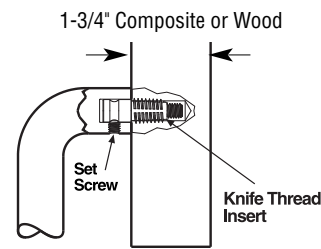
WOOD DOOR - TYPE 8
